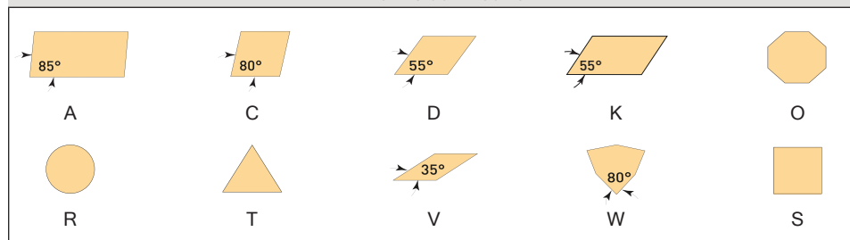
1 - Forma dell'inserto
