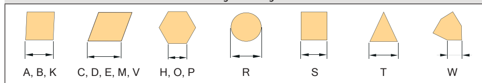
5 - Lunghezza tagliente
